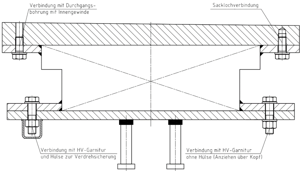
Bild 1: Einbausituationen
